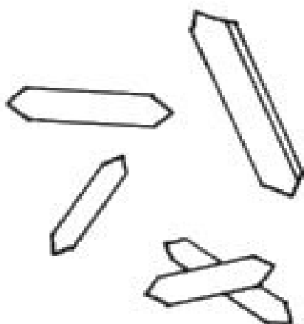
Ácido hipúrico
