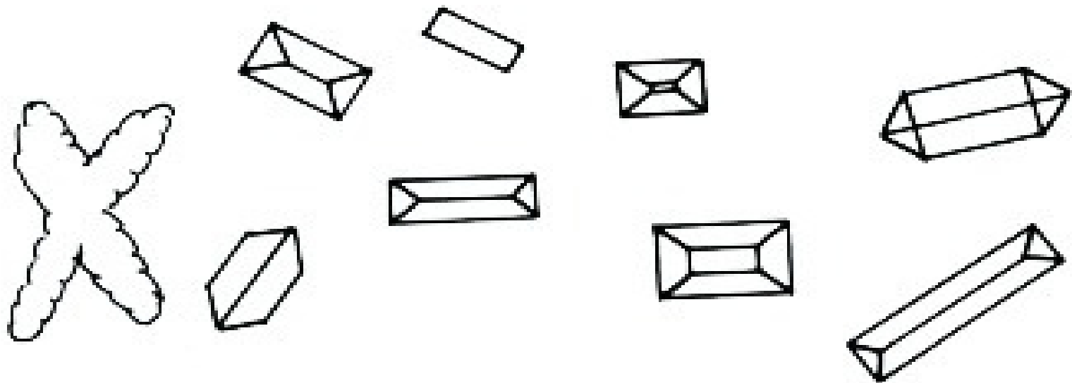
Fosfato triple
