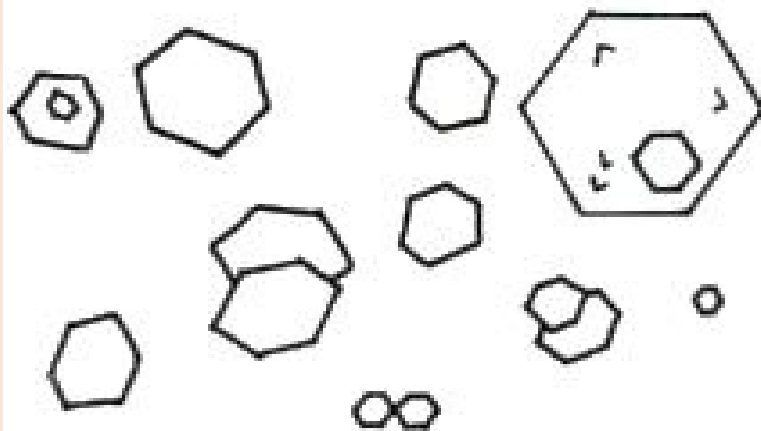
Cistina
