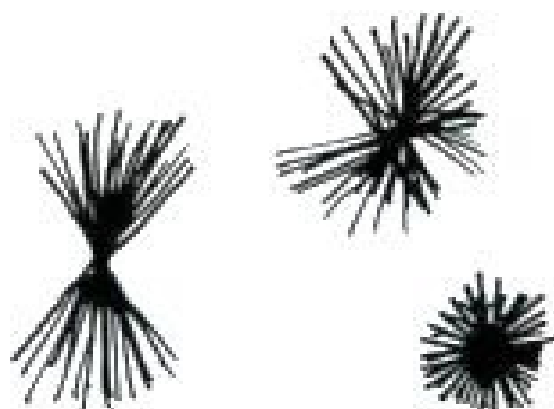
Tirosina
