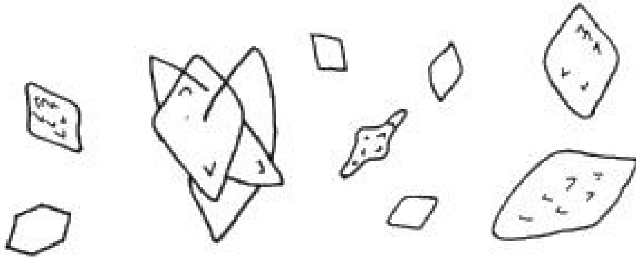
Ácido úrico
